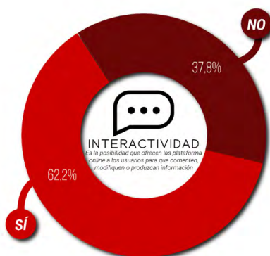
Figura 2. Interactividad
