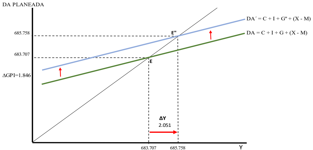
Figura 2. Expansión de la demanda agregada ante un incremento del gasto público.
