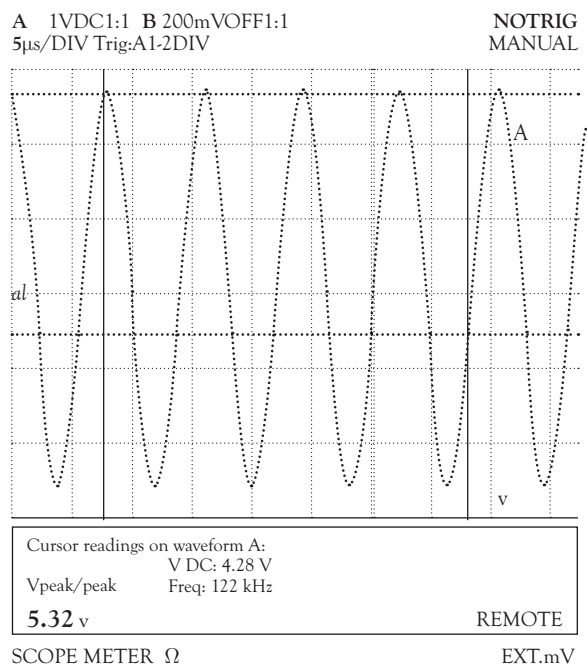
Figura 5. Señal radiada en el shield . Fuente: elaboración propia
