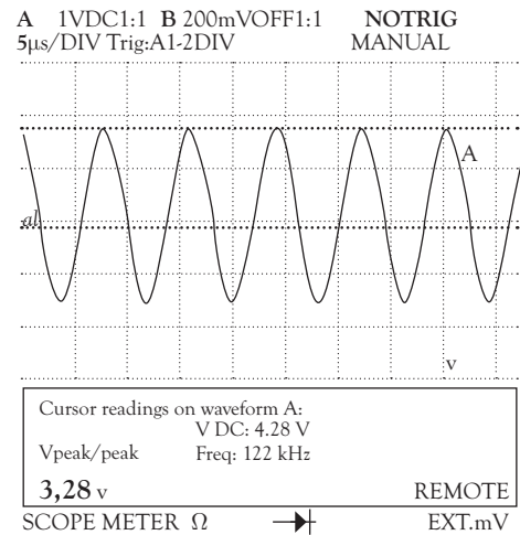
Figura 6. Señal detectada por el shield en presencia de una perturbación. Fuente: elaboración propia
