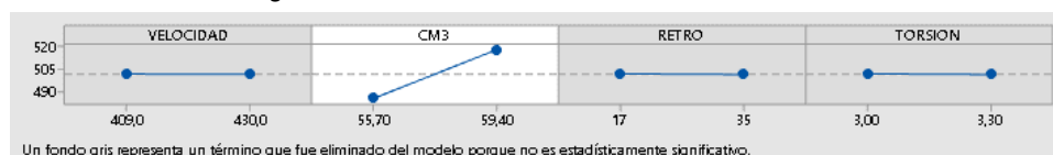
Figura 7. Efectos de los factores en el diseño factorial
